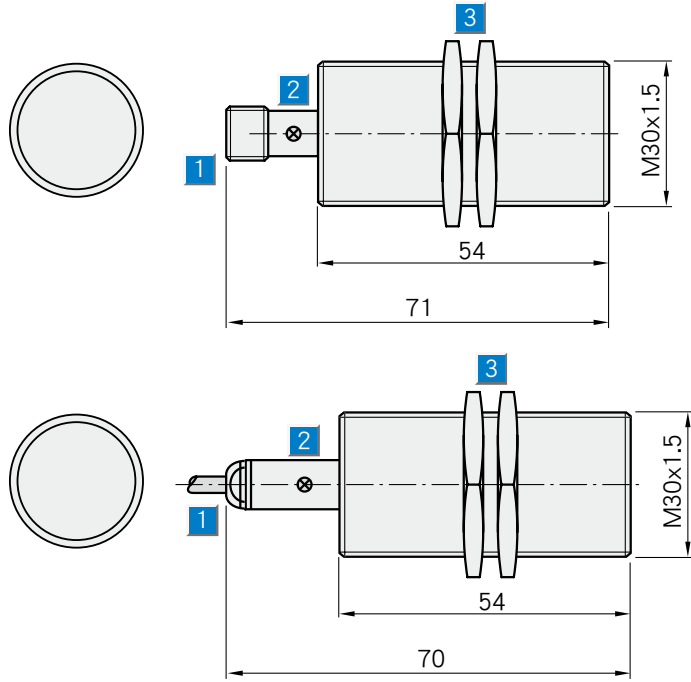
尺寸圖
