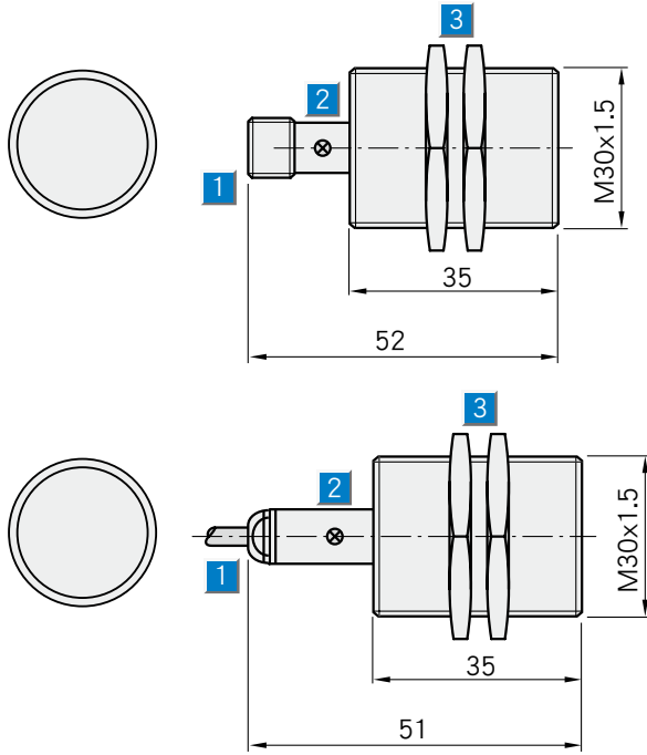
尺寸圖
